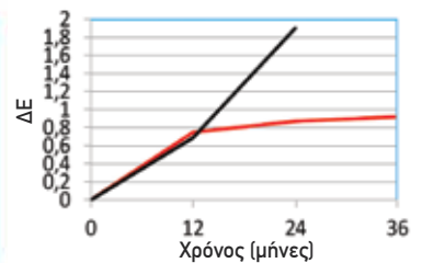
■ Prisma/Ammos* ■ Class1 Διατήρηση απόχρωσης ΔΕ σε συνάρτηση με χρόνο. Χαμηλές τιμές ΔΕ σημαίνουν καλή διατήρηση απόχρωσης *Μέσος όρος των σειρών
